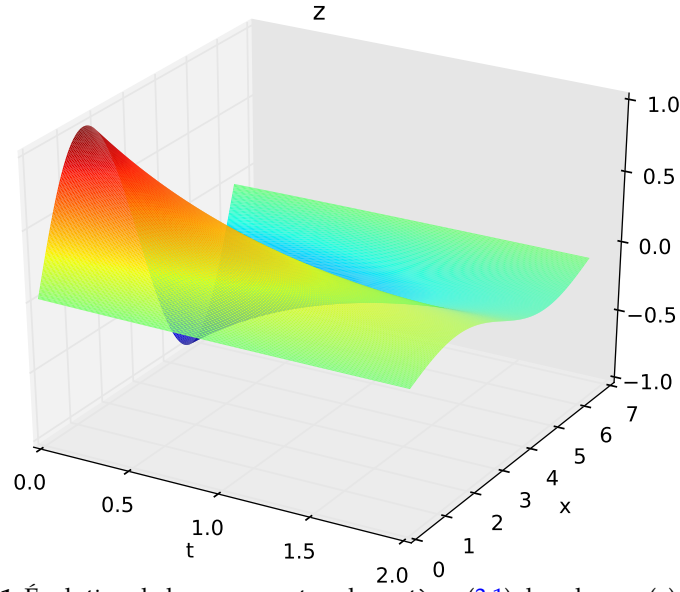
FIGURE V.1: Évolution de la composante z du système (3.1) dans les cas (a) et (b).
