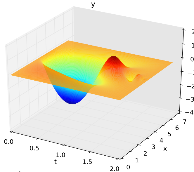
FIGURE V.2: Évolution de la composante y du système (3.1) dans le cas (a).
