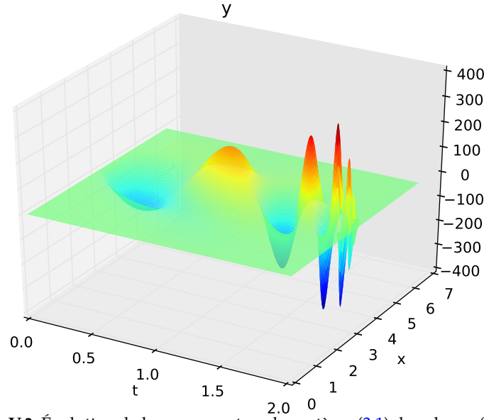
FIGURE V.3: Évolution de la composante y du système (3.1) dans le cas (b).
