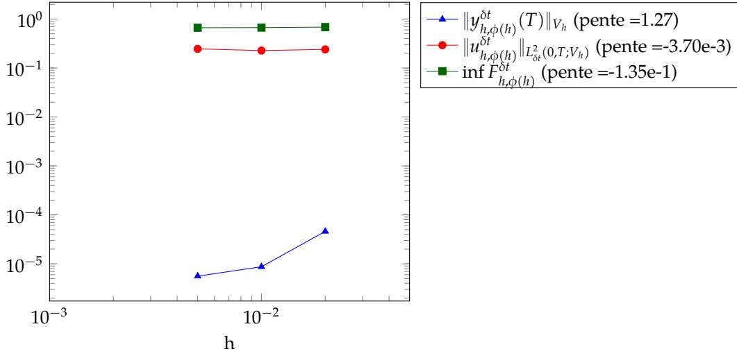
FIGURE V.4: Distance à la cible \|y_{h,\phi(h)}^{\delta t}(T)\|_{V_h} , norme du contrôle \|u_{h,\phi(h)}^{\delta t}\|_{L^2_{\delta t}(0,T;V_h)} et valeur minimale de la fonctionnelle \inf_{L^2_{\delta t}(0,T;V_h)} F_{h,\phi(h)}^{\delta t} dans le cas \alpha(x) = x
